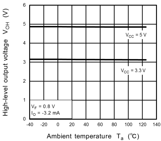
Fig. 13.2.6 V_{OH} - T_a
