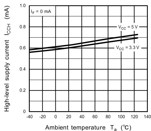
Fig. 13.2.8 I_{CCH} - T_a
