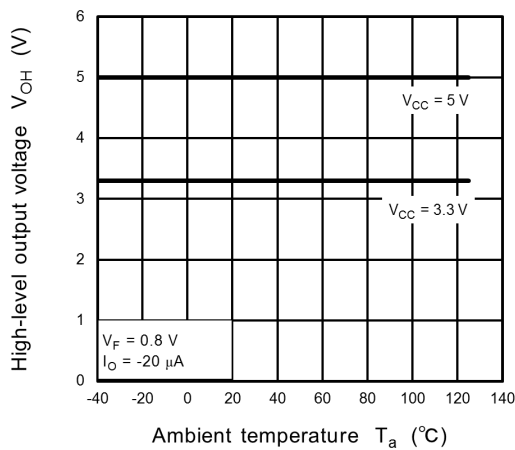
Fig. 13.2.5 V_{OH} - T_a
